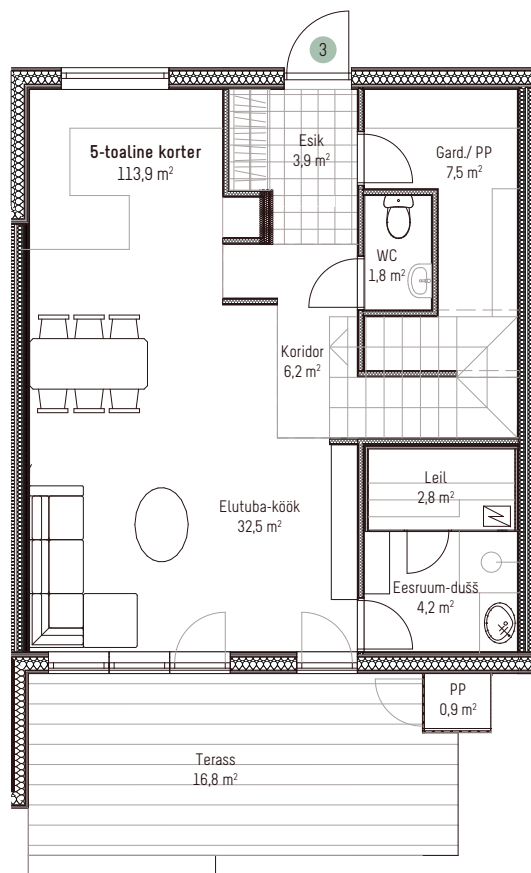
1.korrus
